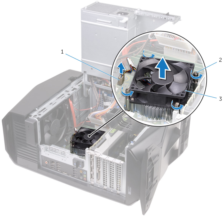
圖 30. 卸下處理器風扇和散熱器組件
