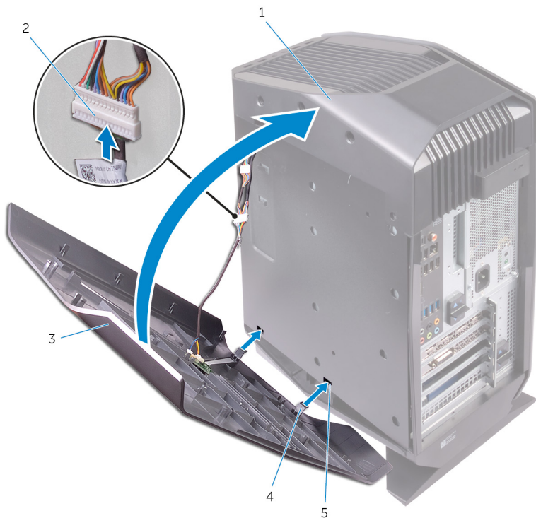
圖 6. 連接指示燈纜線
