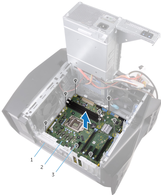
圖 51. 卸下主機板
