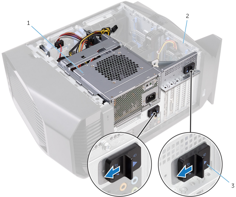
圖 18. 滑動電源供應器固定框架釋放門鎖
