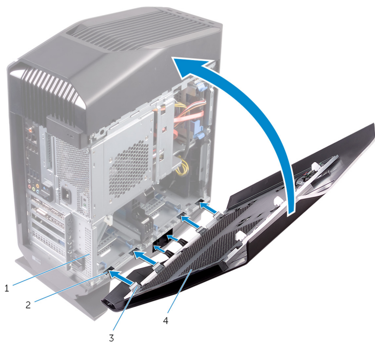
圖 3. 裝回左蓋
