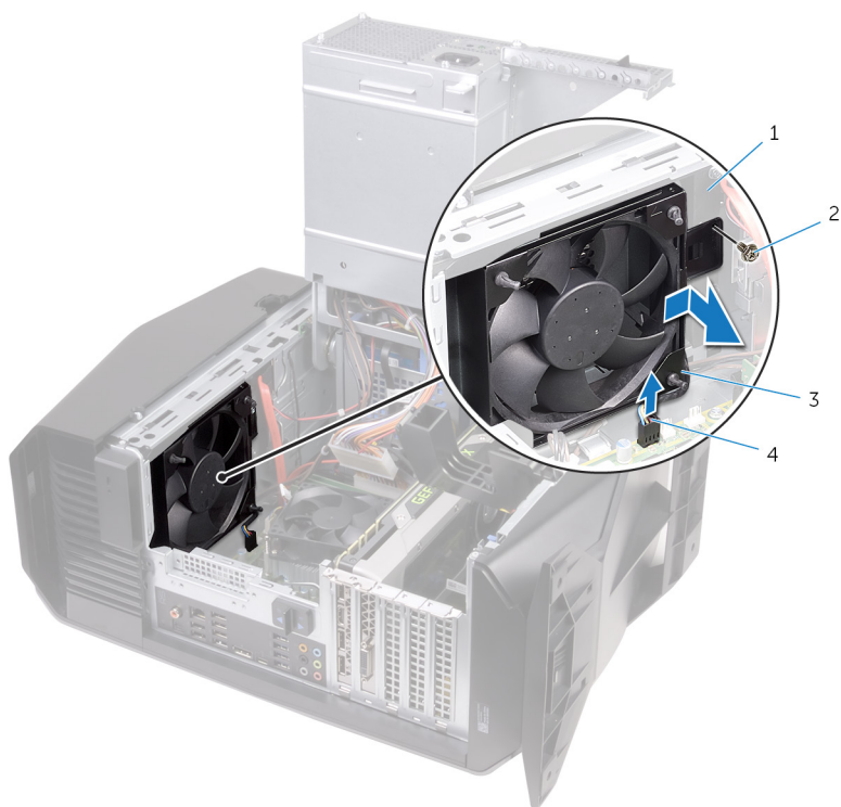
圖 39. 卸下頂部機箱風扇
