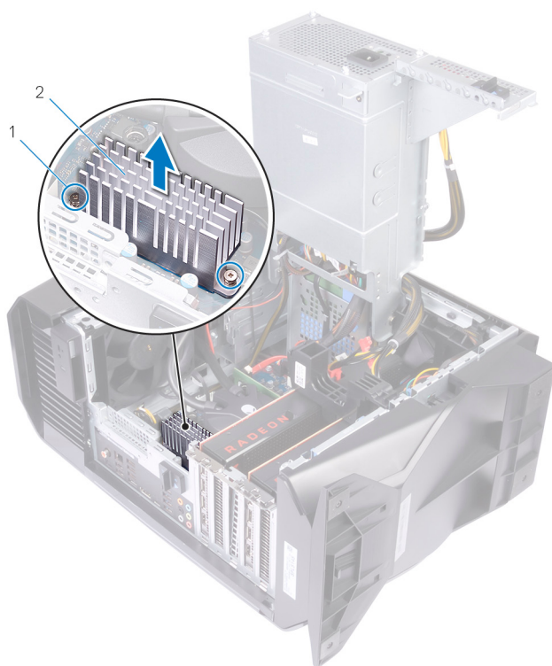
圖 29. 卸下 VR 散熱器
