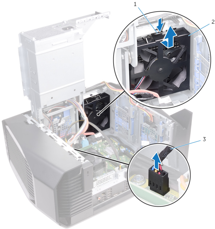
圖 37. 卸下機箱風扇
