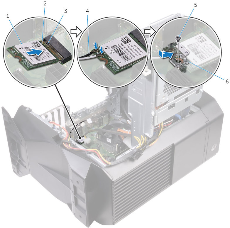
圖 34. 裝回無線網卡
