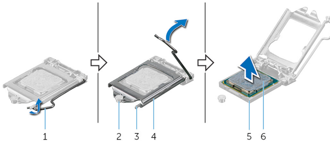
圖 31. 卸下處理器
