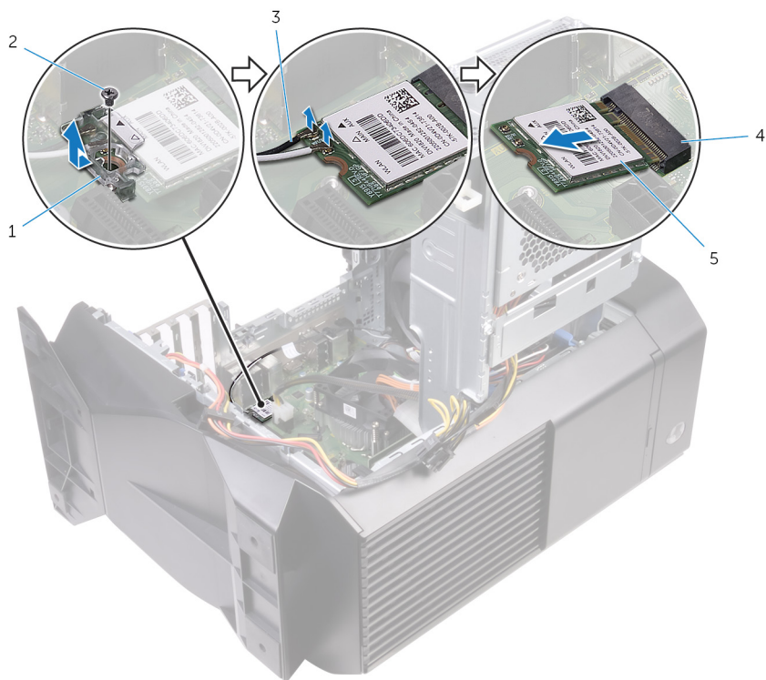
圖 33. 卸下無線網卡
