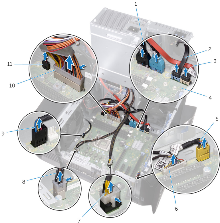
圖 50. 卸下主機板
