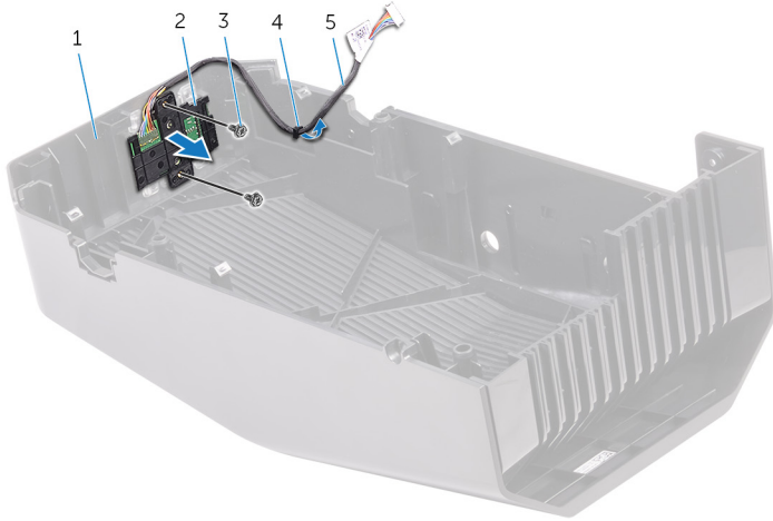
圖 47. 卸下電源按鈕模組
