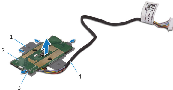
圖 48. 卸下電源按鈕模組
