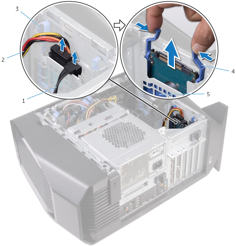
圖 15. 卸下硬碟機
