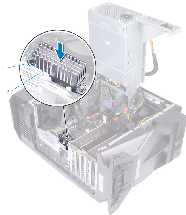
圖 23. 裝回 VR 散熱器
