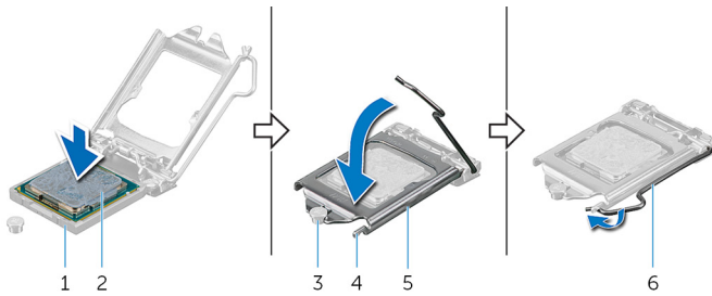
圖 32. 更換處理器
