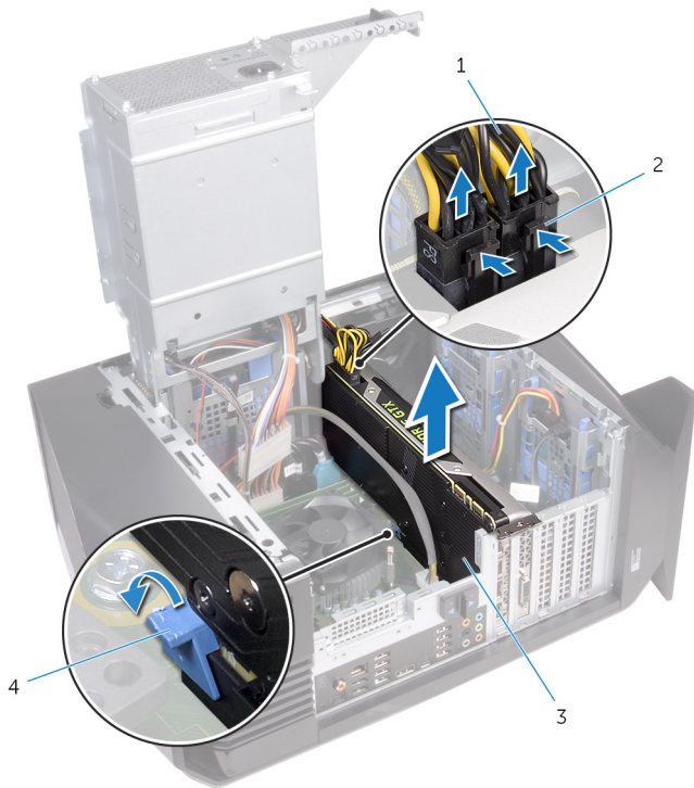
圖 28. 卸下顯示卡
