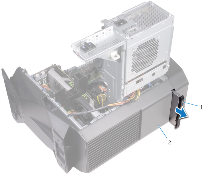
圖 42. 卸下光碟機
