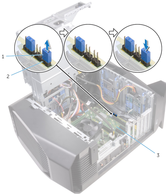
圖 52. 清除忘記的密碼
