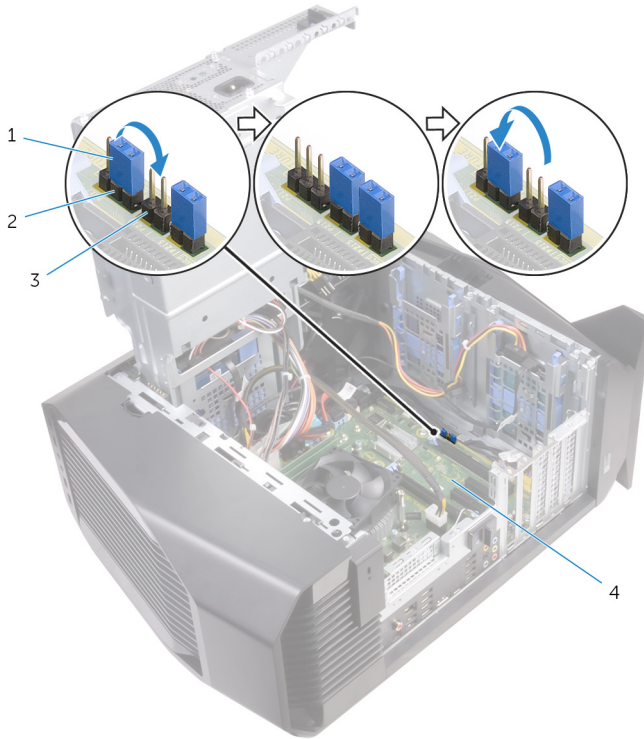
圖 53. 清除 CMOS 設定
