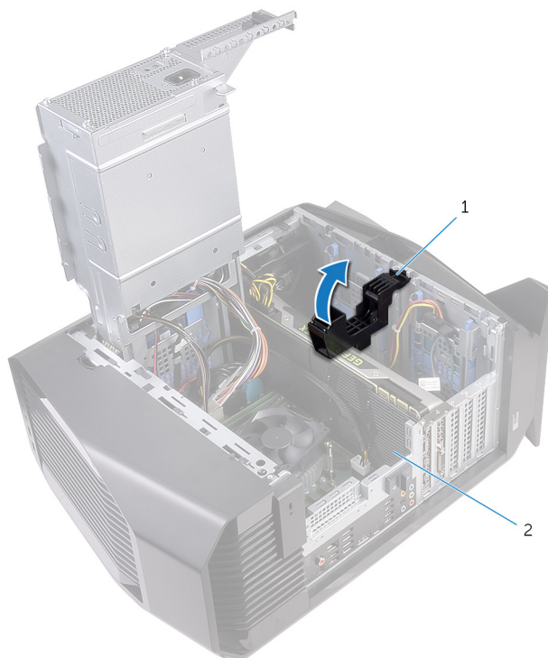
圖 27. 卸下顯示卡
