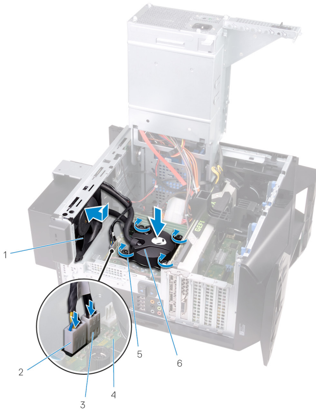
圖 22. 裝回處理器散熱組件
