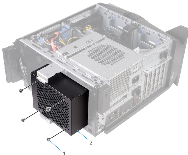
圖 19. 卸下處理器散熱組件
