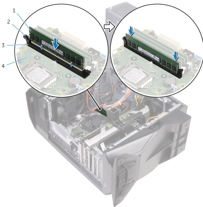
圖 26. 裝回記憶體模組
