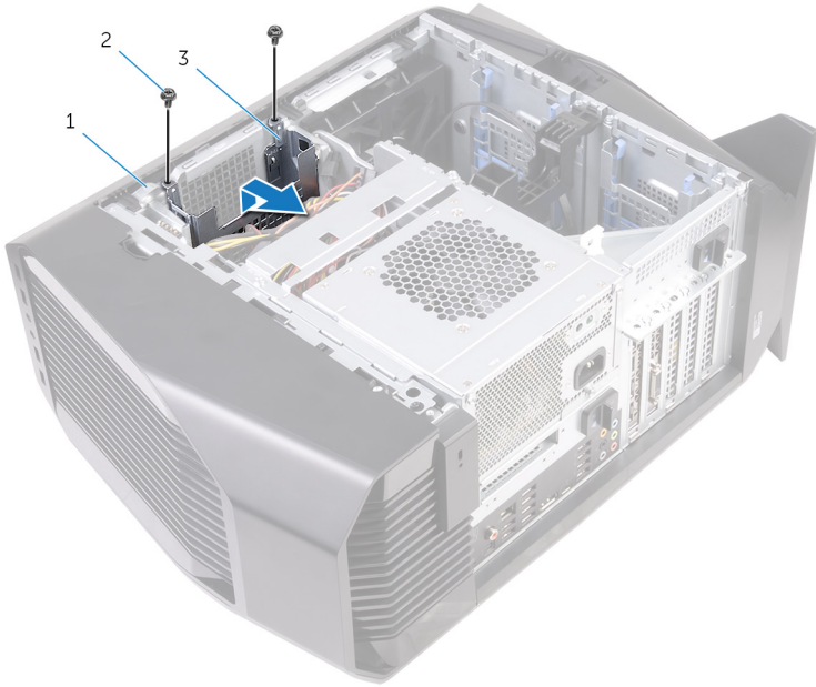
圖 17. 卸下硬碟固定框架
