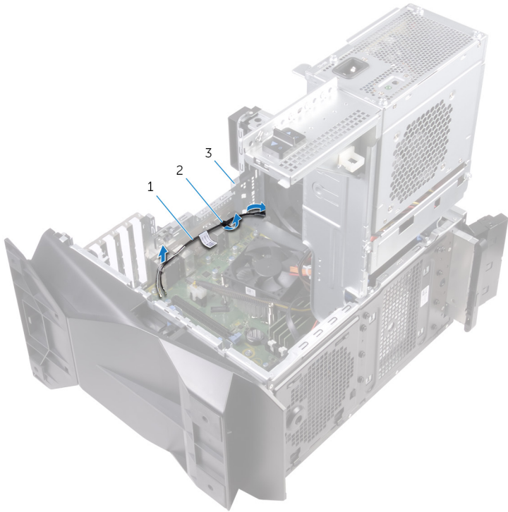
圖 35. 卸下天線纜線
