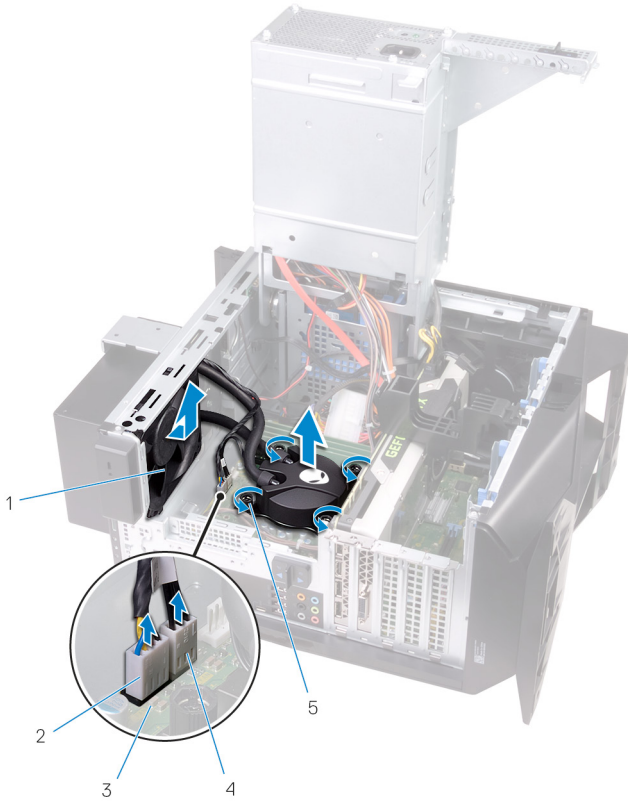
圖 21. 卸下處理器散熱組件
