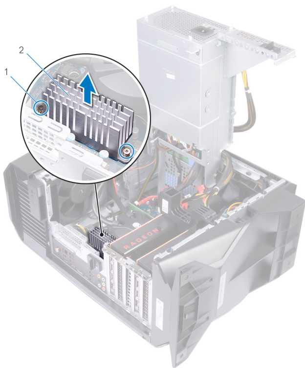
圖 20. 卸下 VR 散熱器
