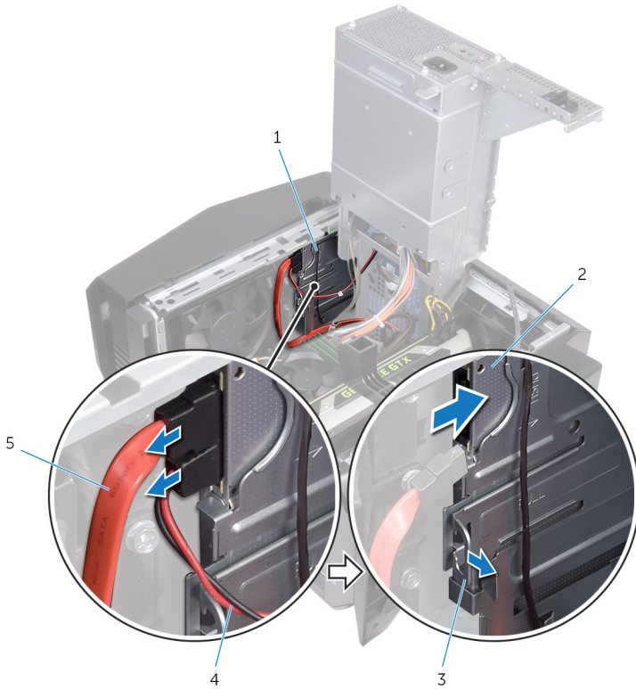
圖 41. 拔下電源線和資料纜線
