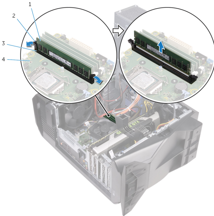
圖 25. 卸下記憶體模組
