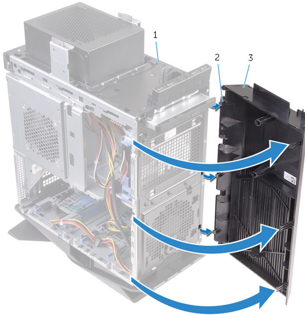
圖 46. 卸下前蓋
